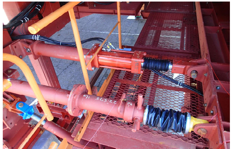
2. 側フォームシリンダー
